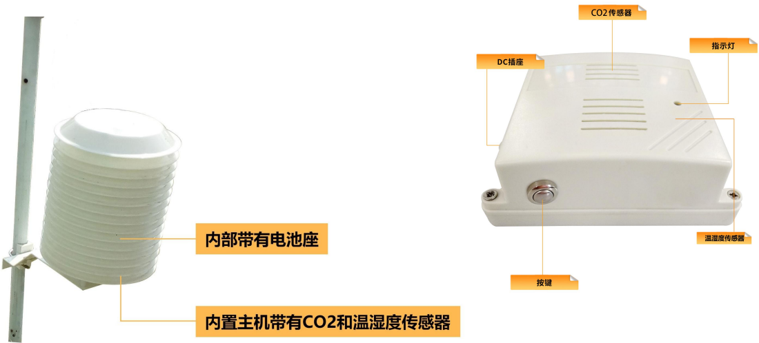
图三 RA0715Y 屏蔽罩内接内接 CO 2 和温湿度 Sensor（以实物为准）
